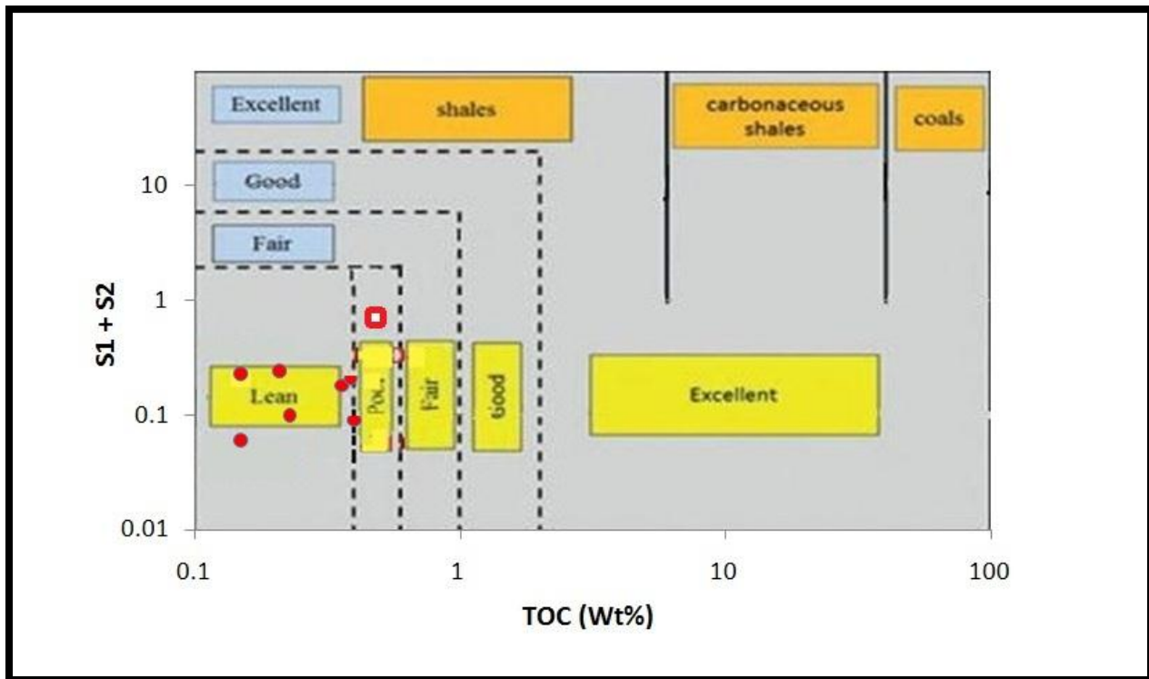
شکل ۴ نمودار تغییرات S1+S2 در برابر TOC بمنظور ارزیابی پتانسیل ژنتیکی نمونه های میوسن جنوب شهرستان ساری (Hung et. al. – 2003) [9]
