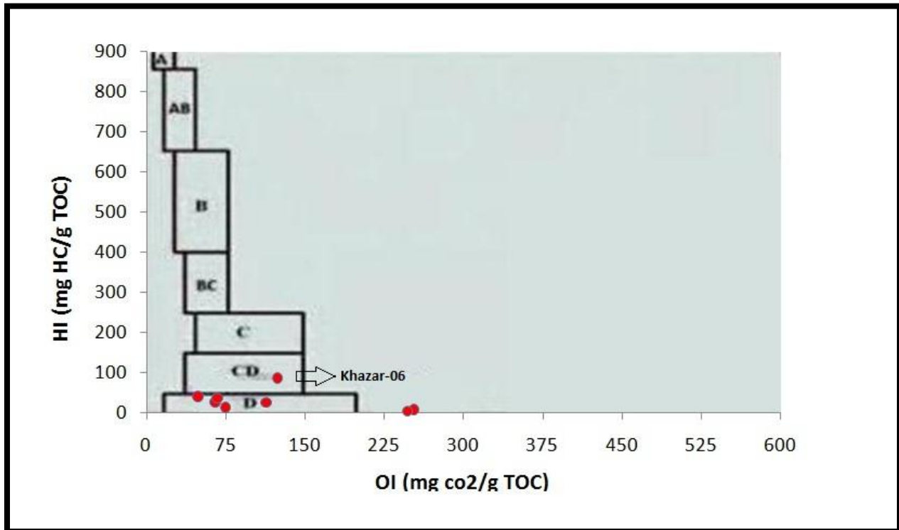
شکل ۷ نمودار تعیین رخساره آلی با استفاده از نسبت تغییرات HI در برابر OI (Jones - 1987) [10]
