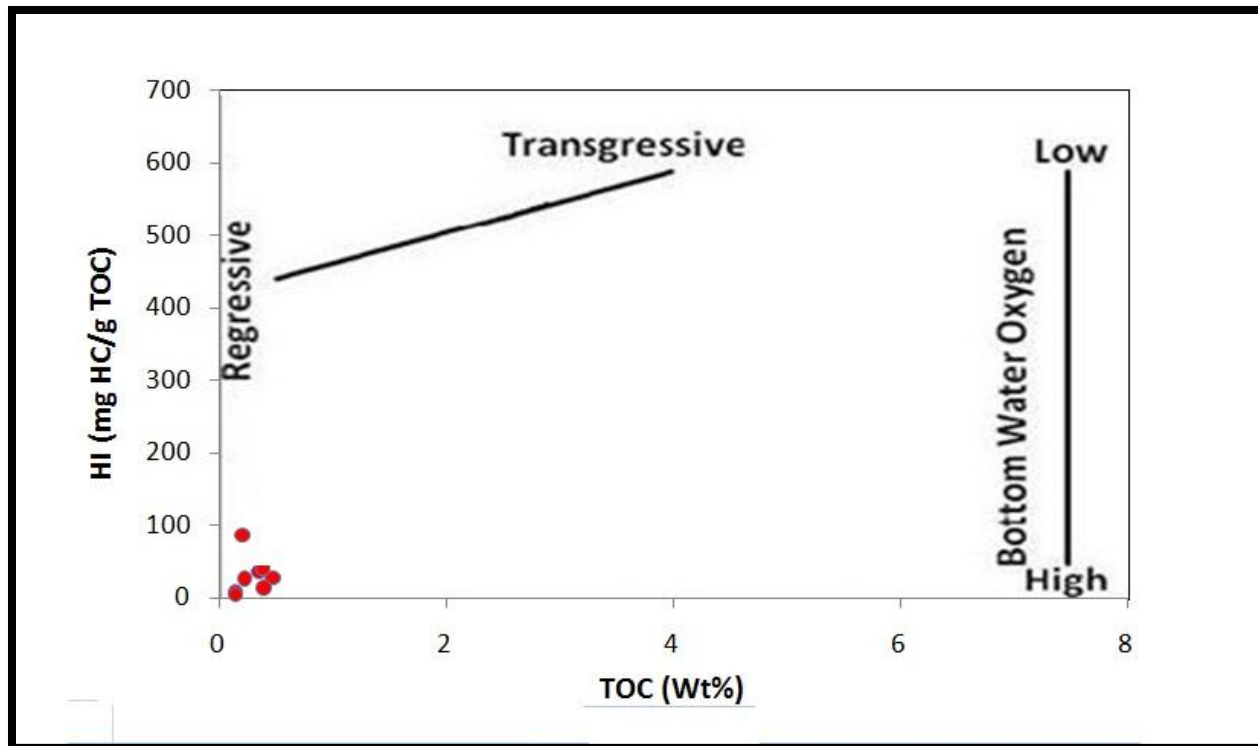
شکل ۸ نمودار مقادیر TOC در مقابل HI بمنظور شناسایی شرایط محیط رسوبگذاری آنها [5] (Dean et. Al. – 1986)
